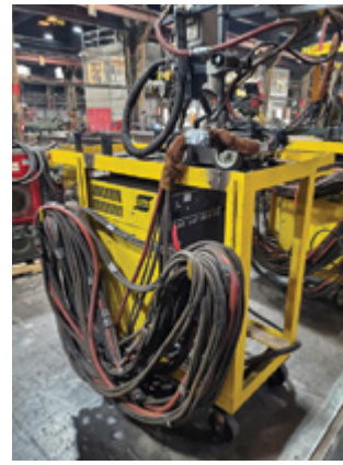
ESAB LAF 1000
